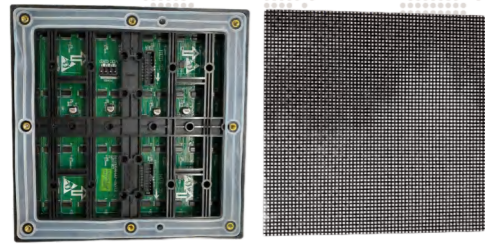
Kích thước mô-đun: 200*200mm
